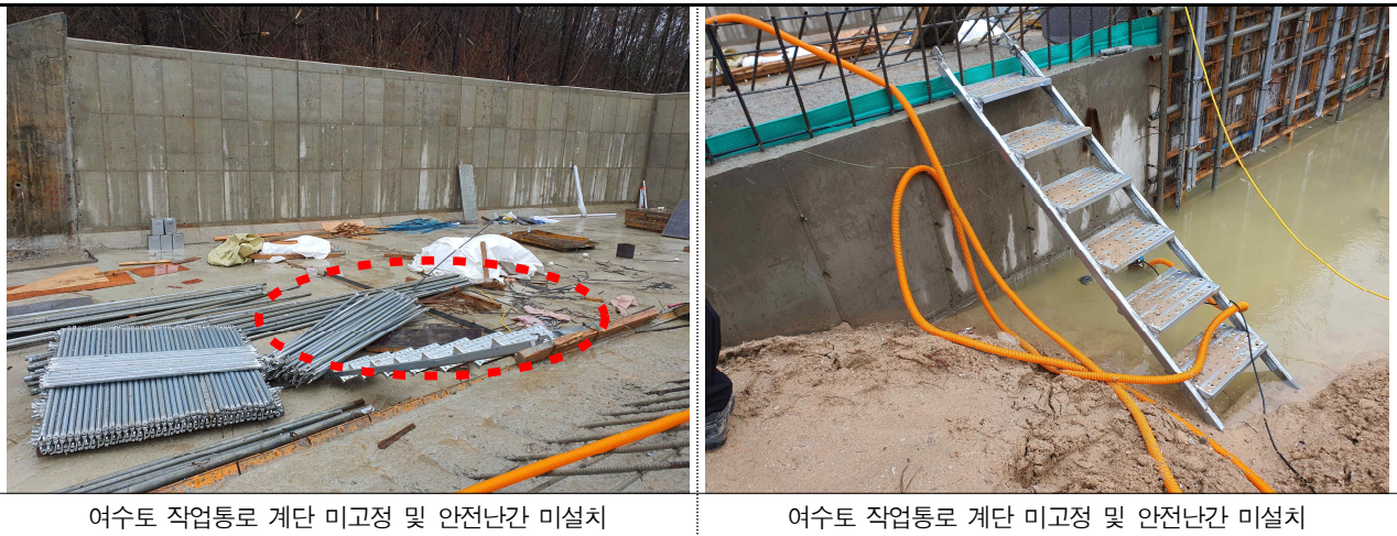
<그림 1> 작업자 통로 계단 안전난간 미설치
